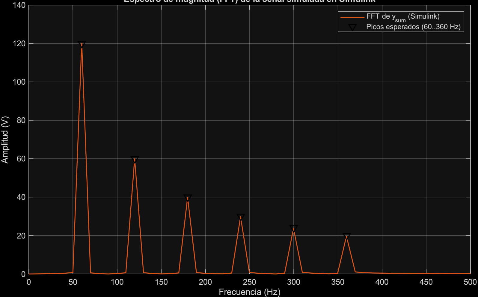
Espectro de magnitud (FFT) de la señal simulada en Simulink
